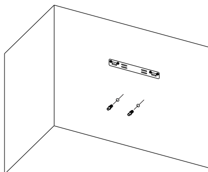
WYWIERĆ OTWORY I WŁÓŻ KOŁKI ROZPOROWE
