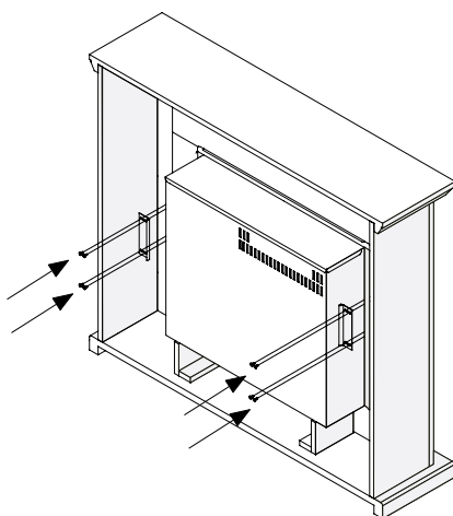
VERWENDEN SIE 8 SCHRAUBEN DES TYPs ST3,5 X 12
